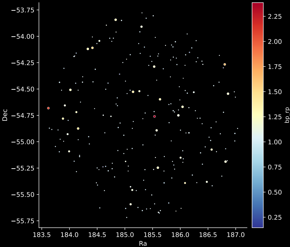
GALAH DR4 Field: [7218] Stars: 224
