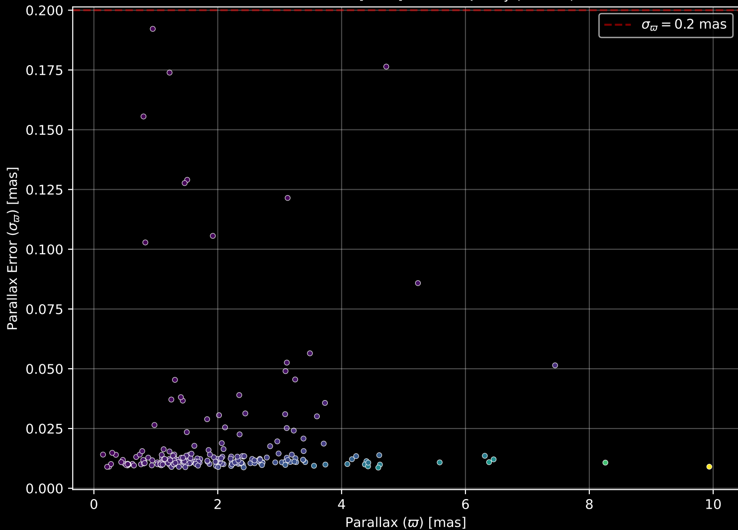
GALAH DR4 Field: [7218] Parallax Quality (n= 224)
