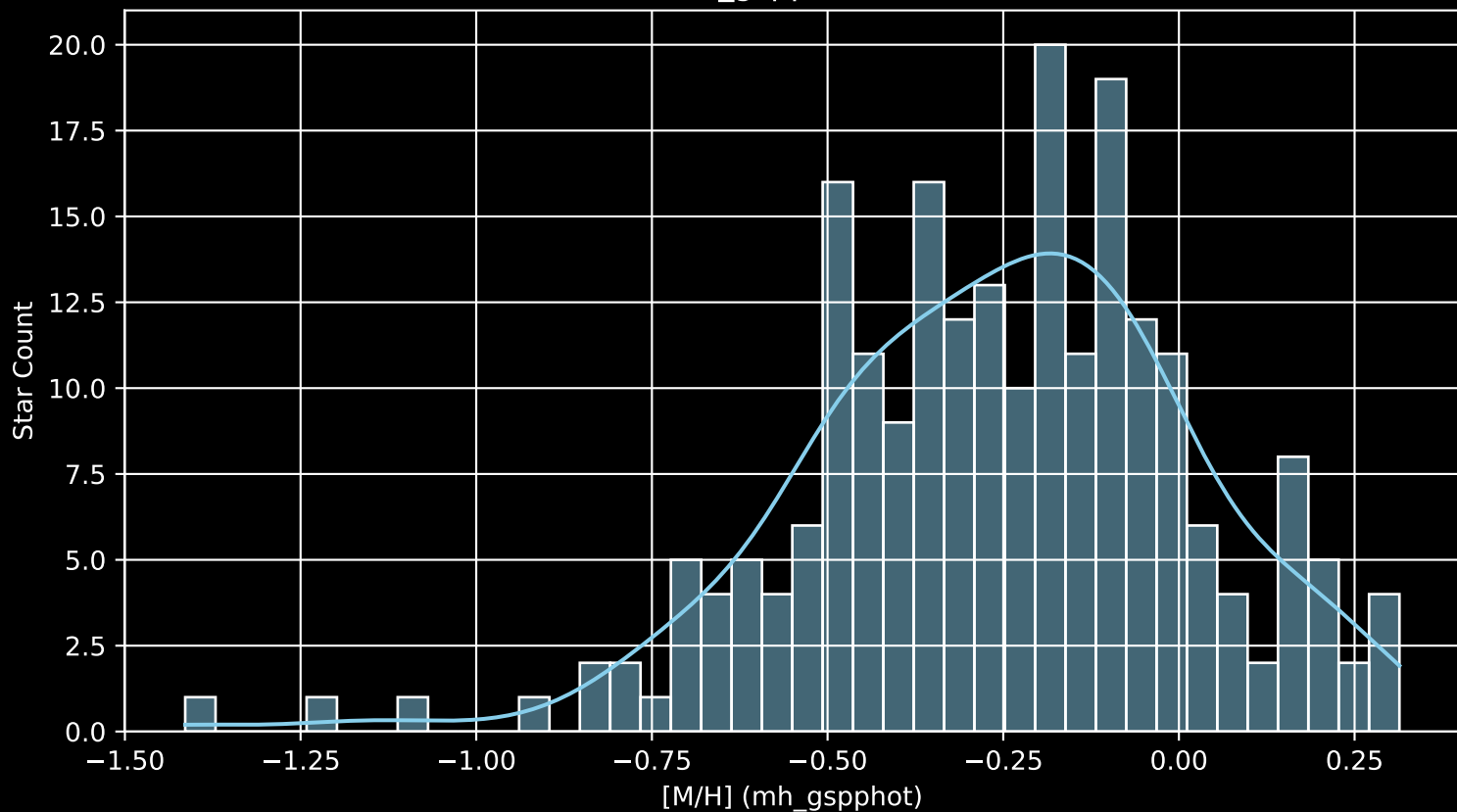
GALAH DR4 Field: [7218] [M/H] (mh_gspphot) (n= 224)
