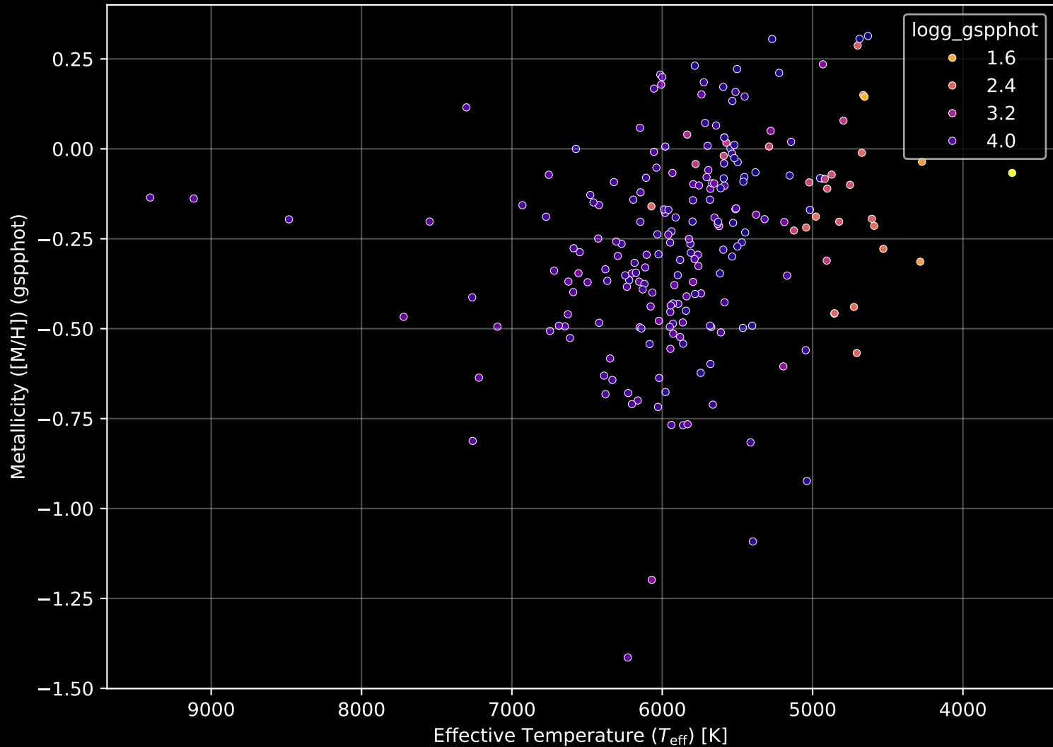
GALAH DR4 Field: [7218] Stellar Population Parameters (n= 224)
